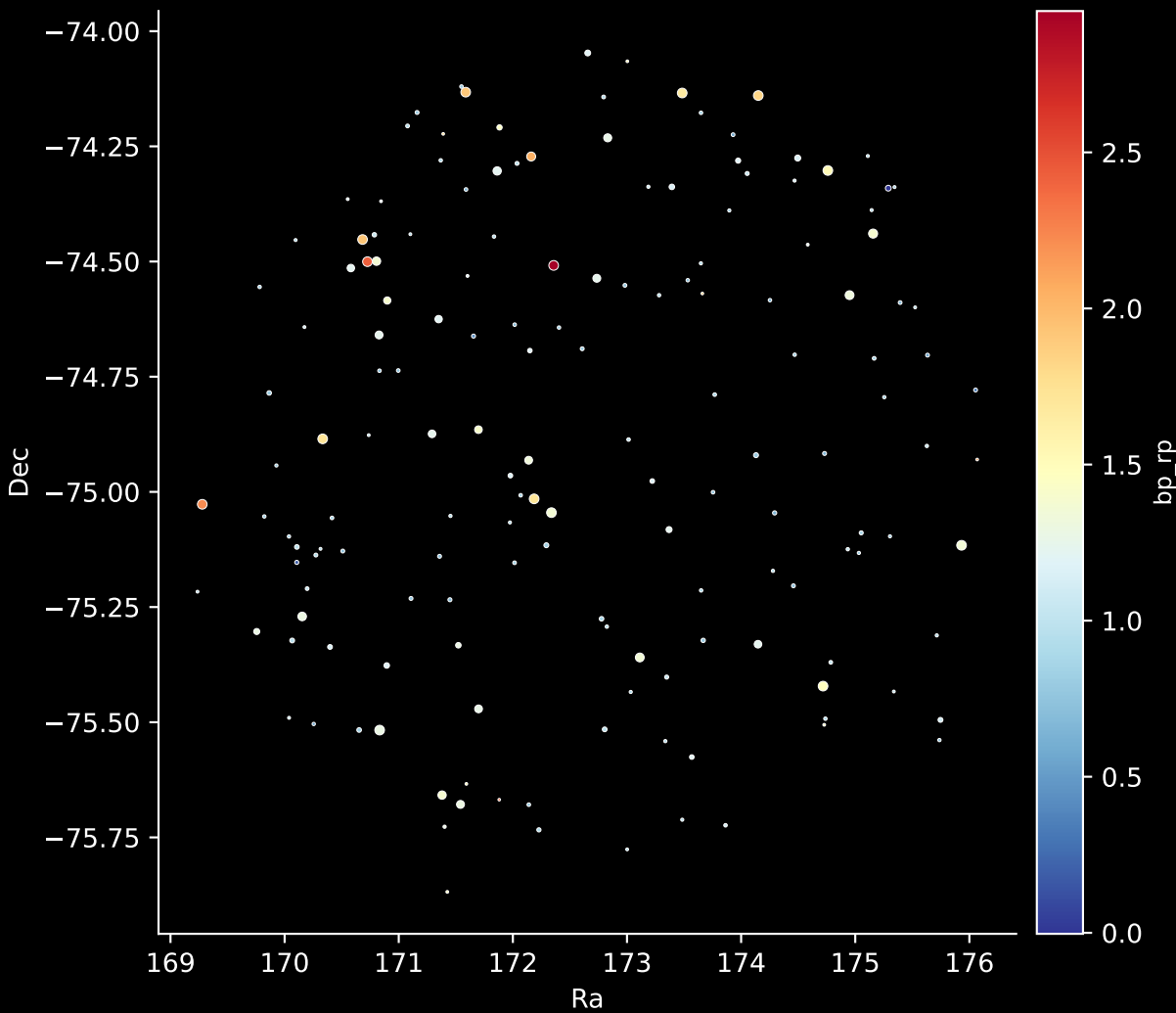
APOGEE DR17 Field: [287-34-O_TESS] Stars: 159
