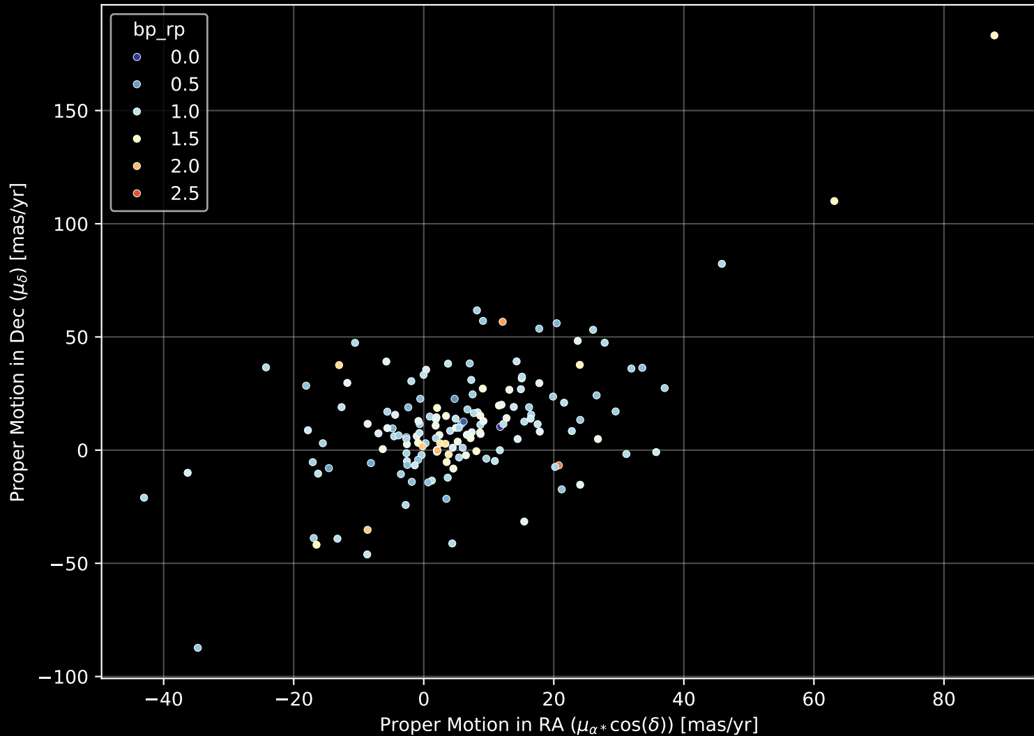
APOGEE DR17 Field: [287-34-O_TESS] Proper Motion Diagram (n= 159)
