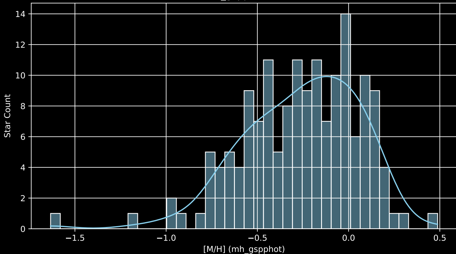
APOGEE DR17 Field: [287-34-O_TESS [M/H] (mh_gspphot) (n= 158)
