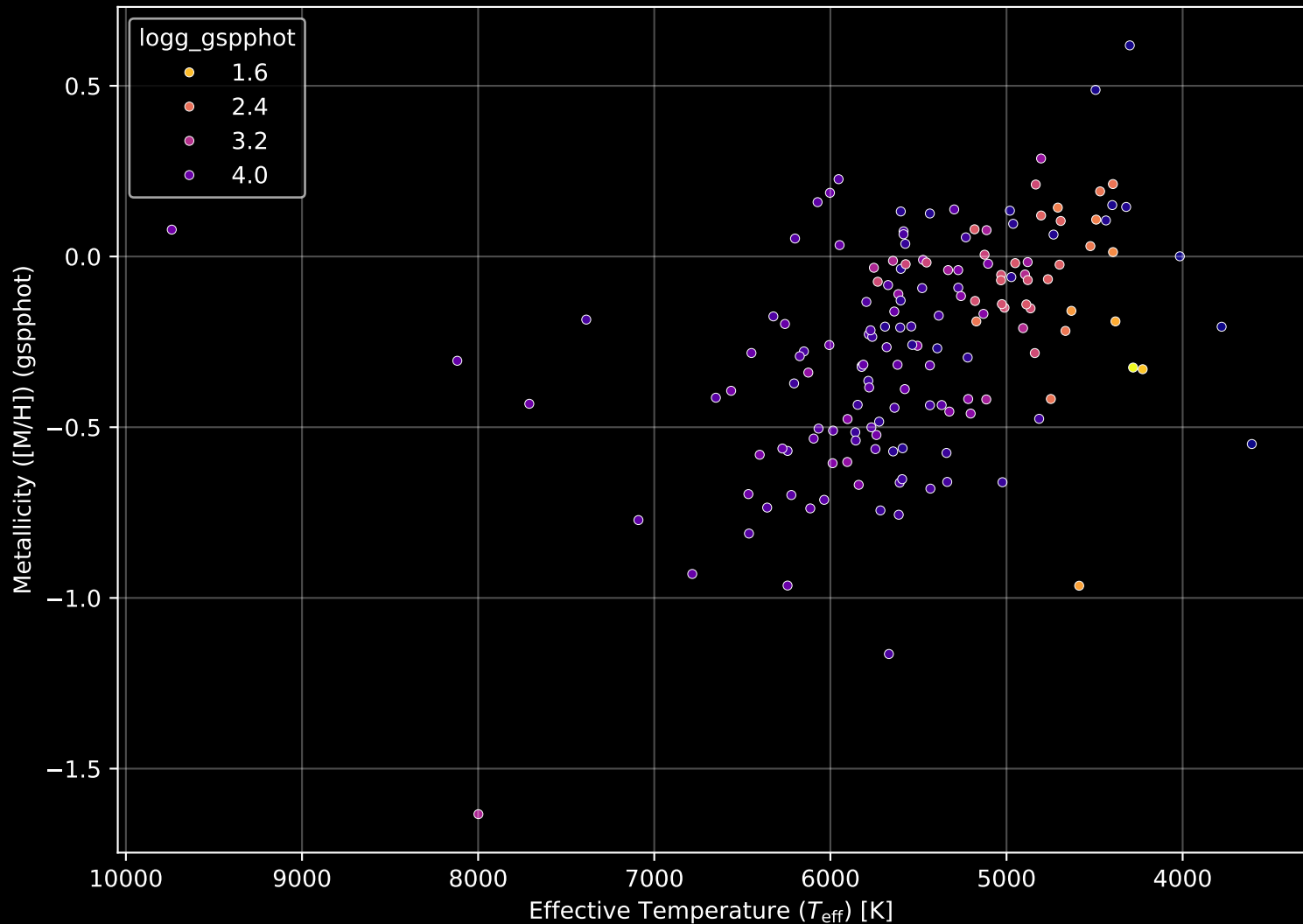
APOGEE DR17 Field: [287-34-O_TESS] Stellar Population Parameters (n= 159)
